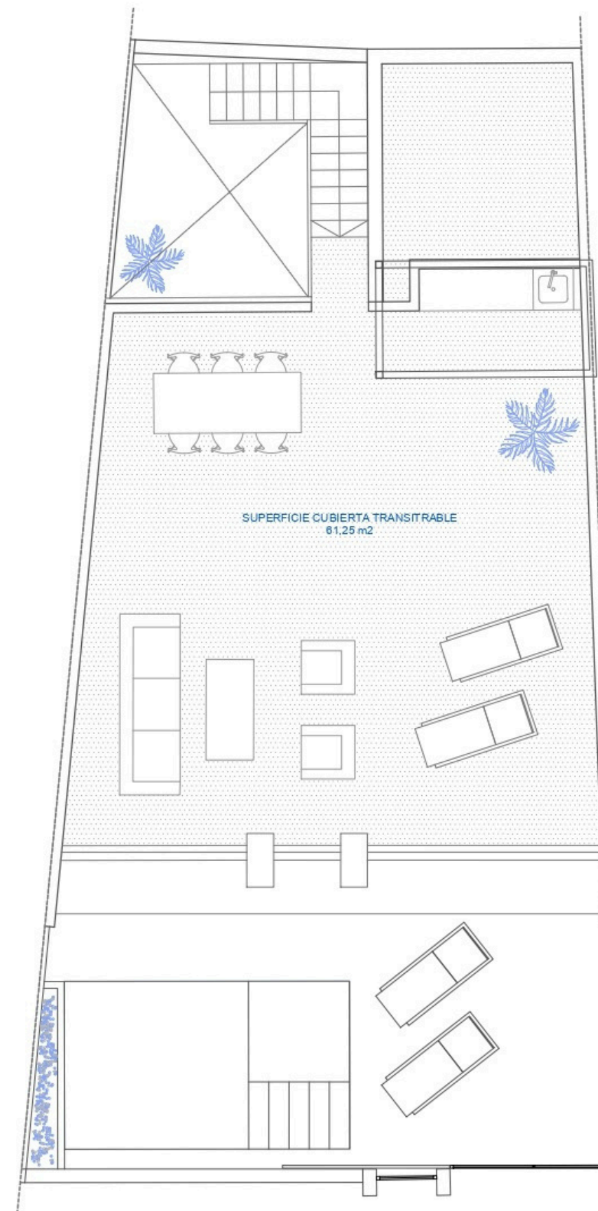
PLANTA SOLARIUM
