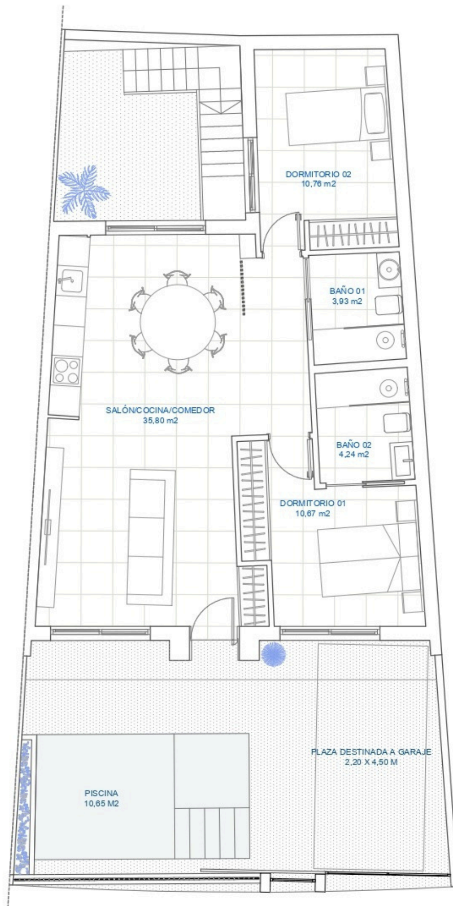
PLANTA BAJA
