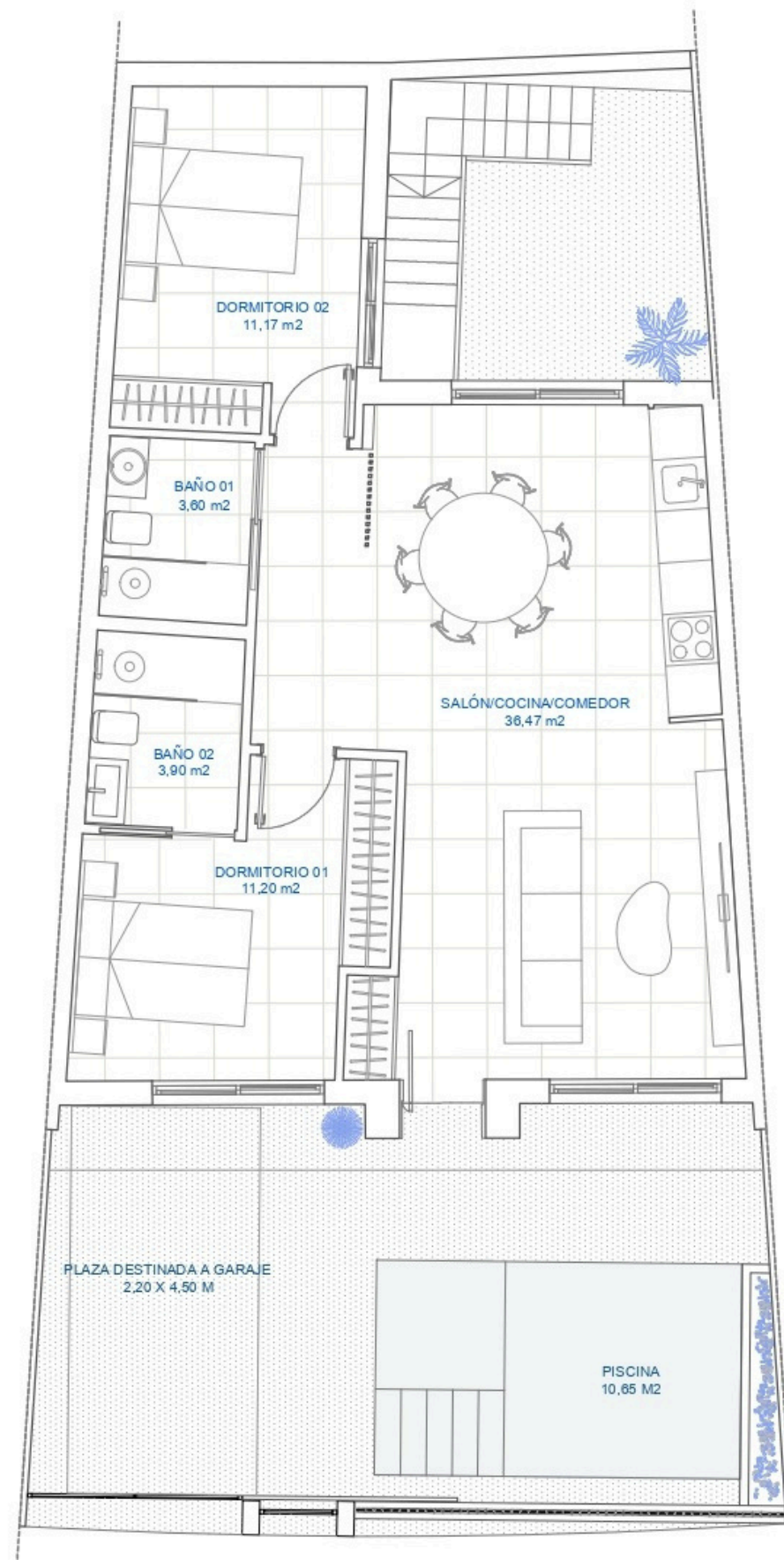
PLANTA BAJA
