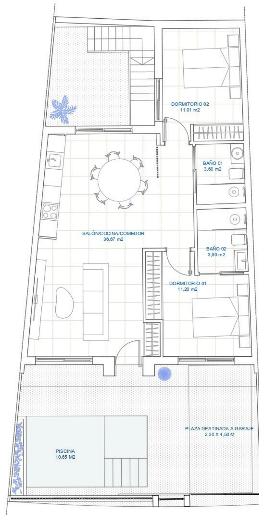
PLANTA BAJA
